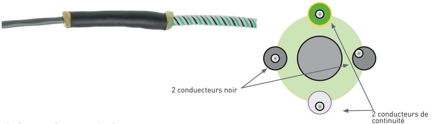
Câble détecteur FG-ACS en coupe avec ses quatre conducteurs
