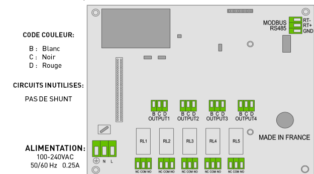
Schéma de câblage FG-ALS4-OD
