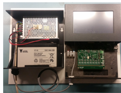
Exemple de connexion entre le BATTERY BACKUP et la centrale FG-NET
