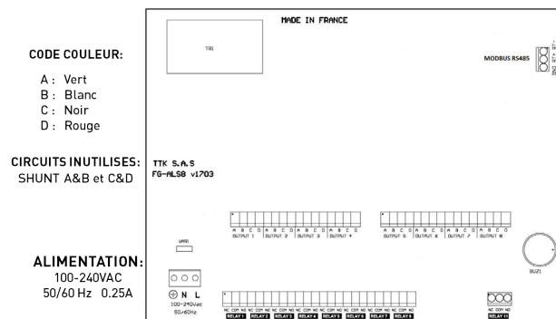
Schéma de câblage FG-ALS8
