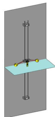
Système de flottaison à guidage mural
