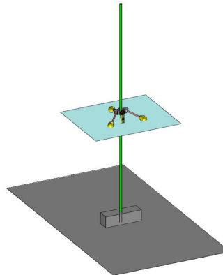
Système de flottaison guidé par des barres
