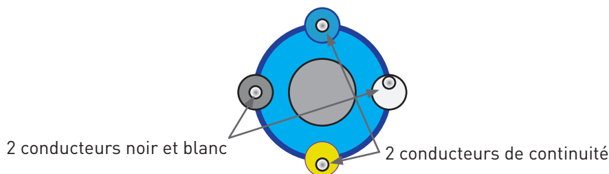
Câble détecteur FG-ECS en coupe avec ses quatre conducteurs
