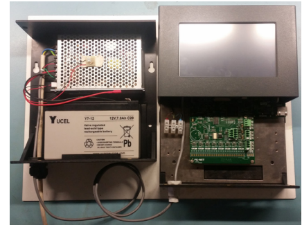
Exemple de connexion entre le BATTERY BACKUP et la centrale FG-NET
