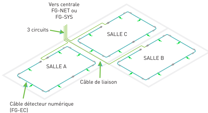
Figure 1.5 Installation « horizontale »
