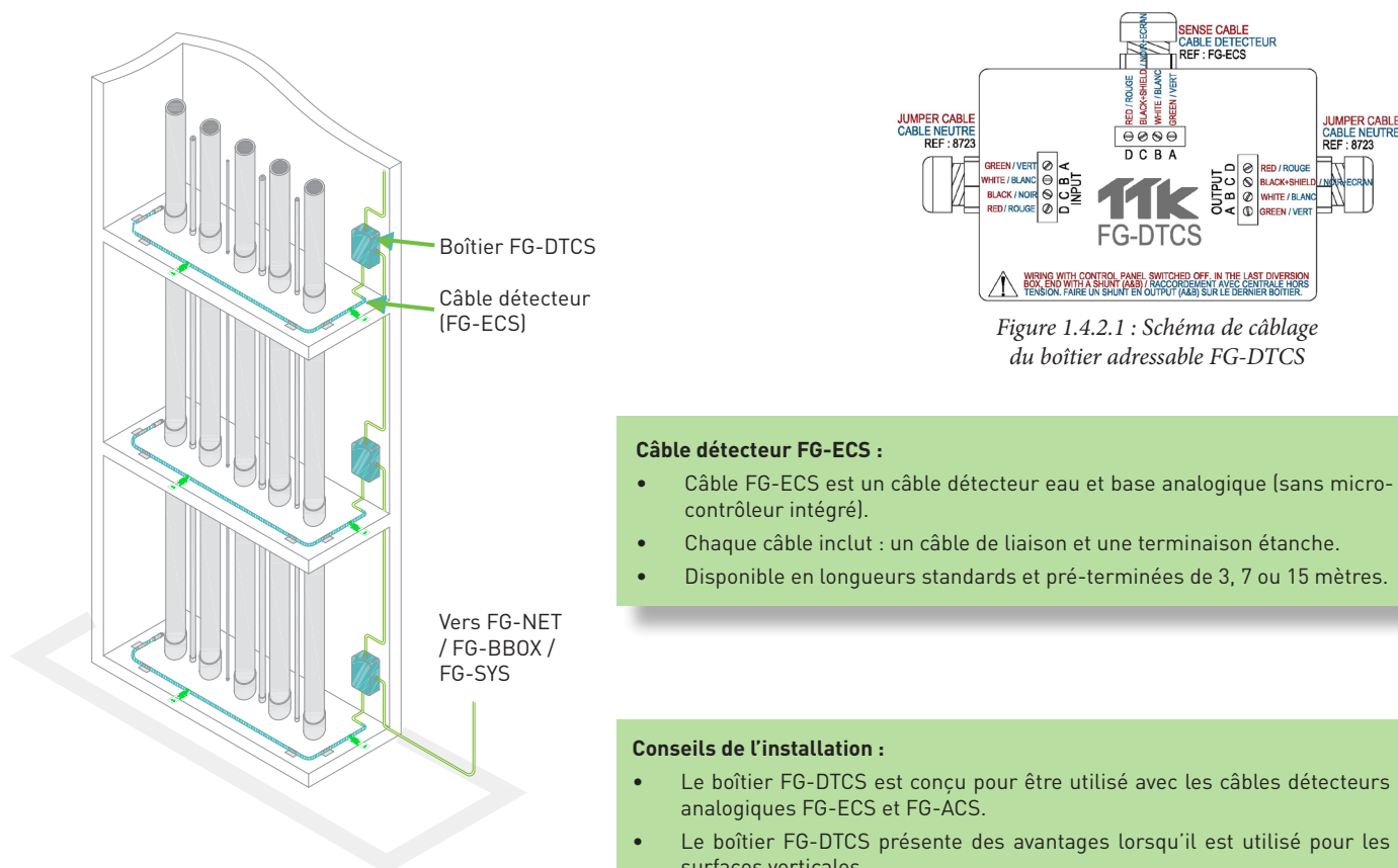
Figure 1.4.2 : Installation avec boîtiers adressables FG-DTCS
