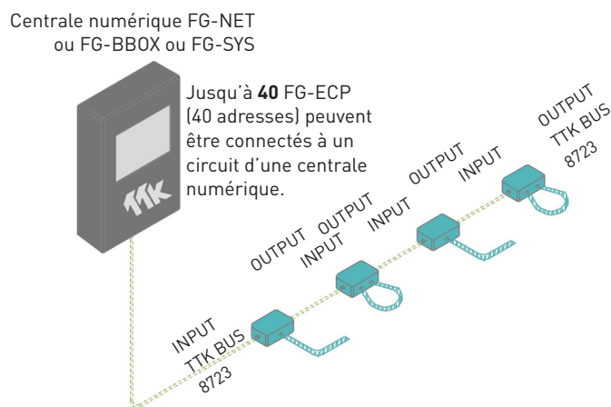
Figure 1.3.1: Installation de FG-ECP avec FG-NET
