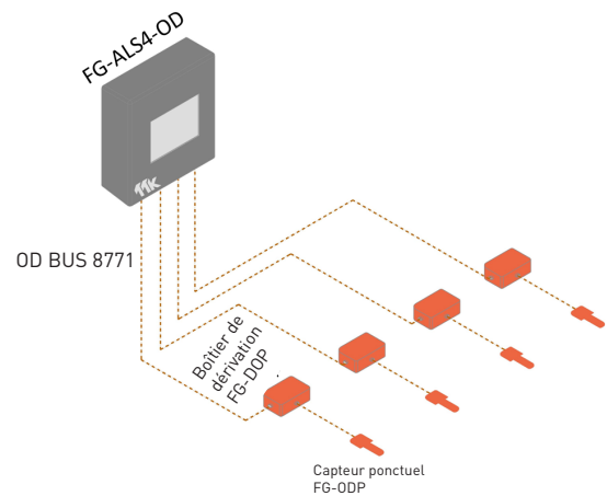
Figure 1.3.2.1: Installation du capteur ponctuel FG-ODP sur 4 circuits de la centrale FG-ALS4-OD utilisant boîtier FG-DOP
