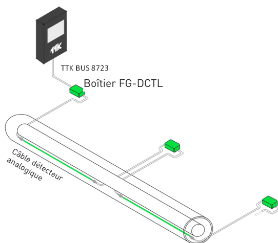
Figure 1.4.4 : Installation avec boîtier d'interface FG-DCTL
