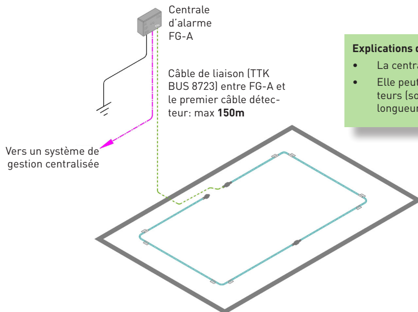
Figure 1.2.8 Installation avec FG-A
