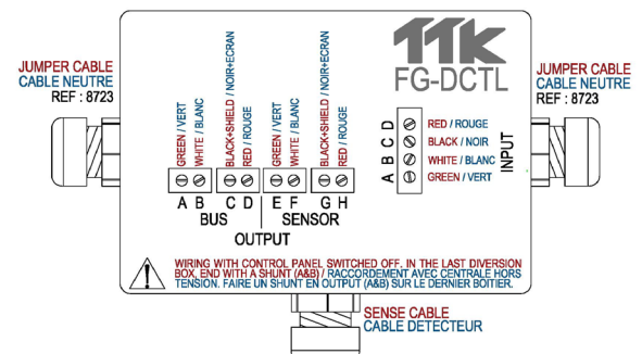
Figure 1.4.4.1: Schéma de câblage du boîtier d'interface FG-DCTL
