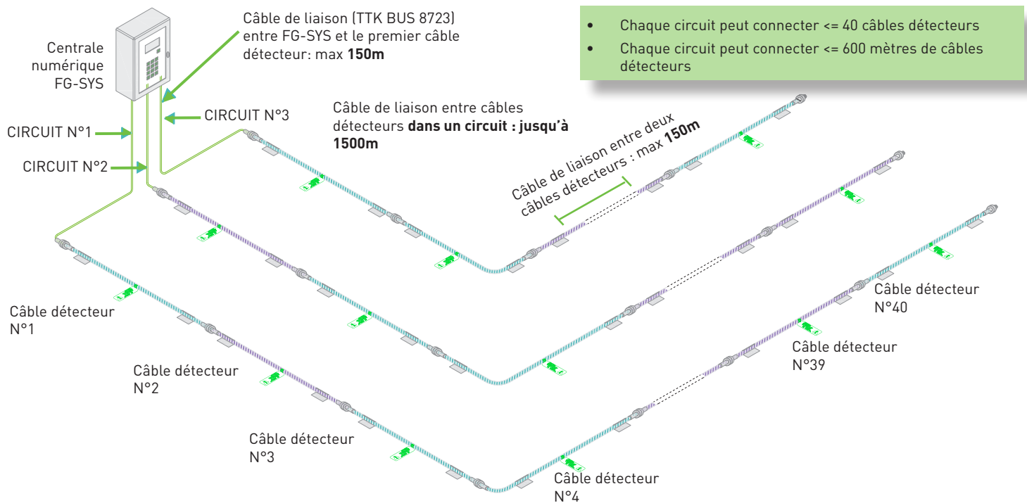
Figure 1.2.2 Installation basique du FG-SYS avec 3 circuits
