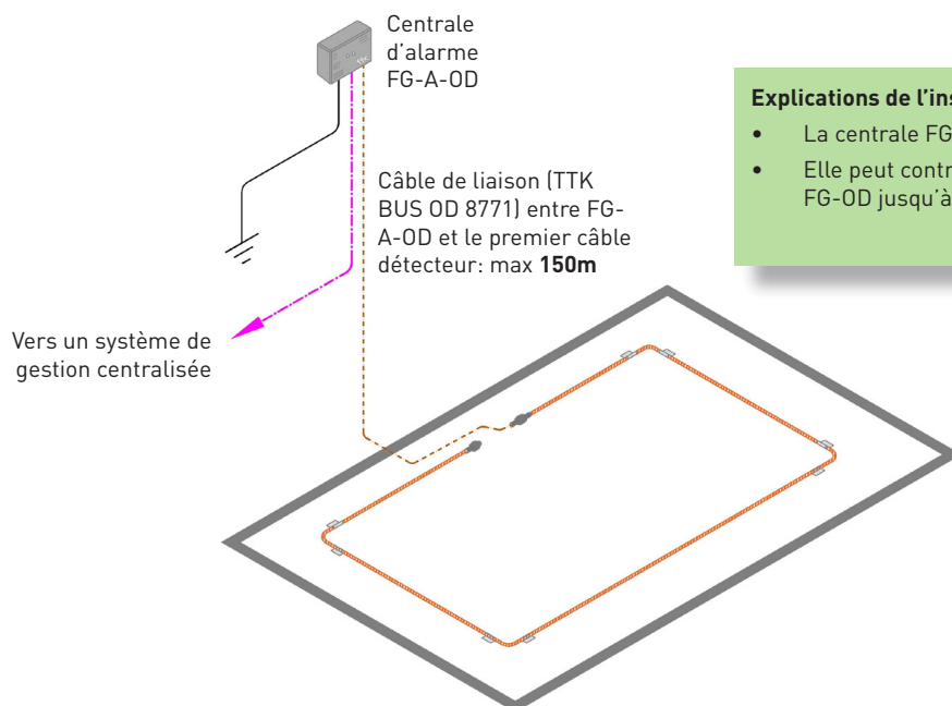
Figure 1.2.9 Installation avec FG-A-OD
