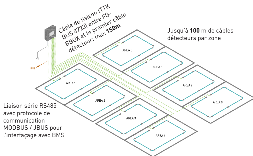
Figure 1.2.4 : Installation de FG-ALS8 avec 8 zones
