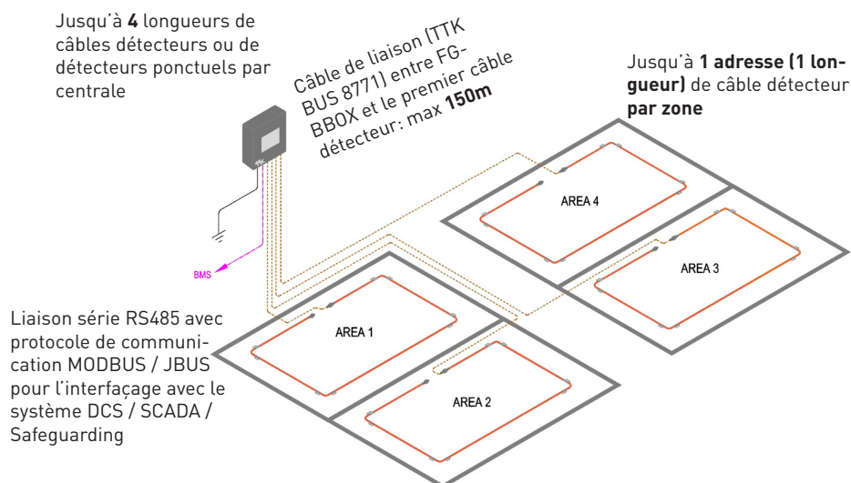
Figure 1.2.7 : Installation de FG-ALS4-OD avec 4 zones
