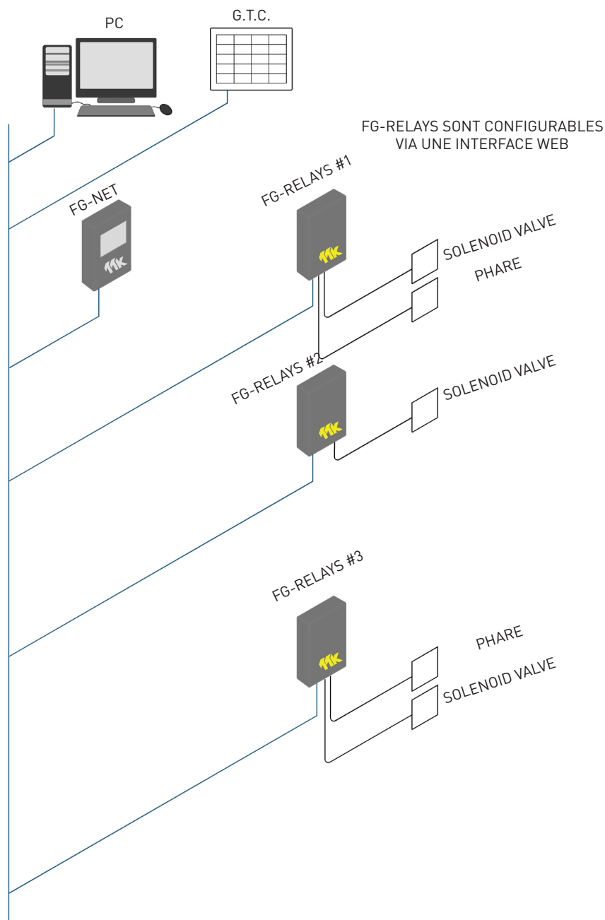
Figures 1.8 la connexion de FG-RELAYS, FG-NET et G.T.C.
