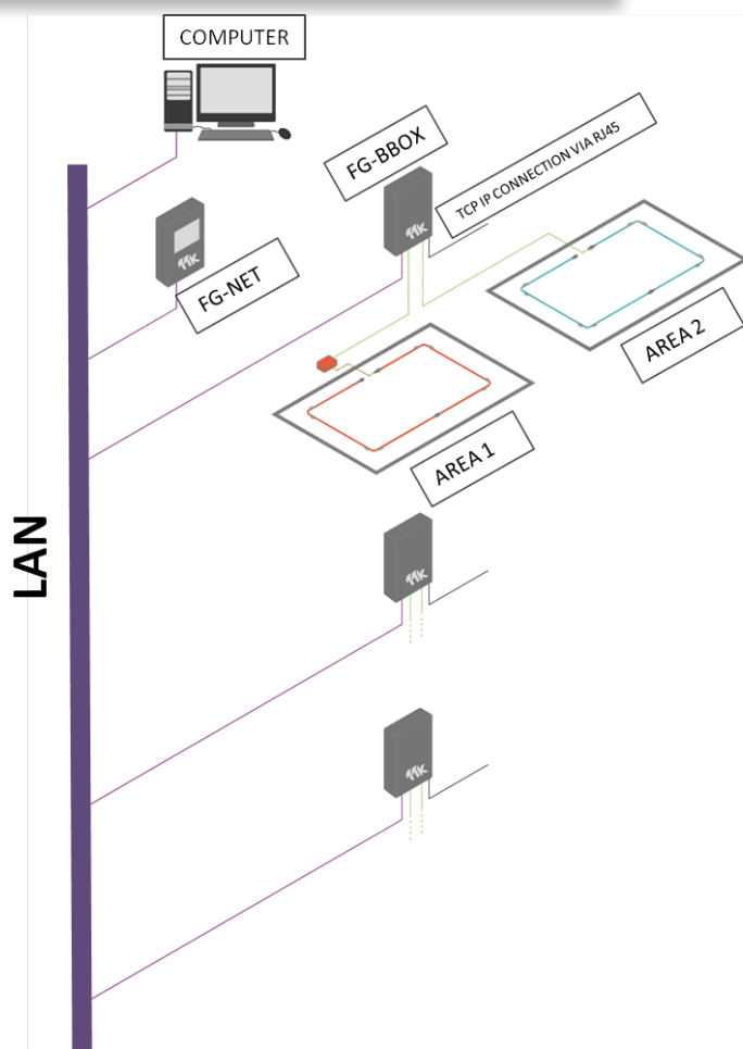
Figures 1.2.3.1 Connexion FG-BBOX avec FG-NET sur réseau Ethernet
