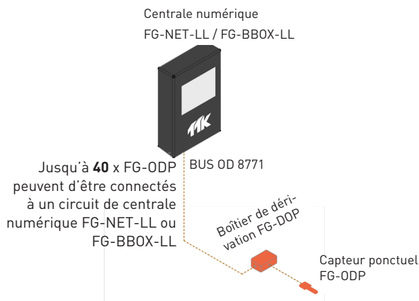
Figure 1.3.2: Installation du capteur ponctuel FG-ODP avec 1 circuit de la centrale numérique FG-NET-LL utilisant boîtier FG-DOP
