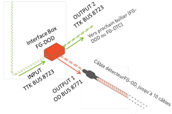
Figure 1.4.5.1: Connexion du boîtier d'interface FG-DOD
