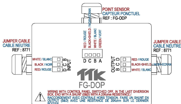
Figure 1.4.6 : Schéma de câblage du boîtier de dérivation du capteur ponctuel FG-DOP
