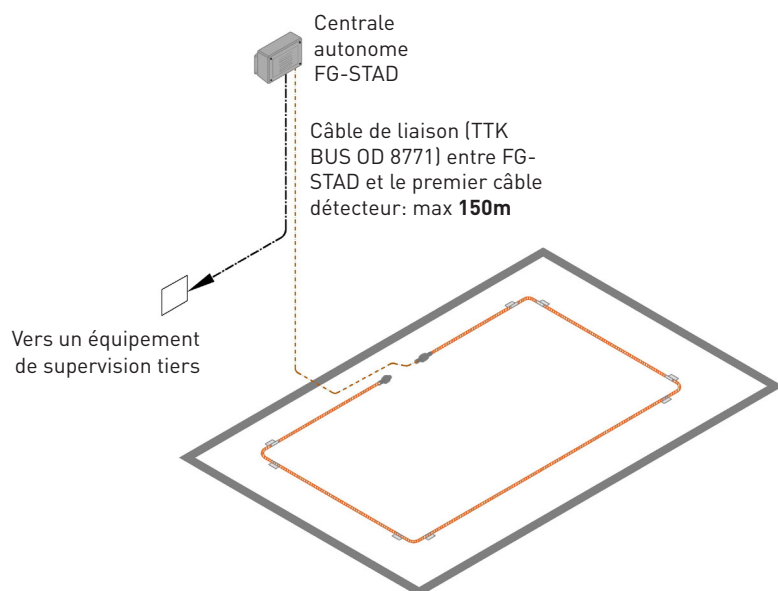
Figure 1.2.10 Installation avec FG-STAD
