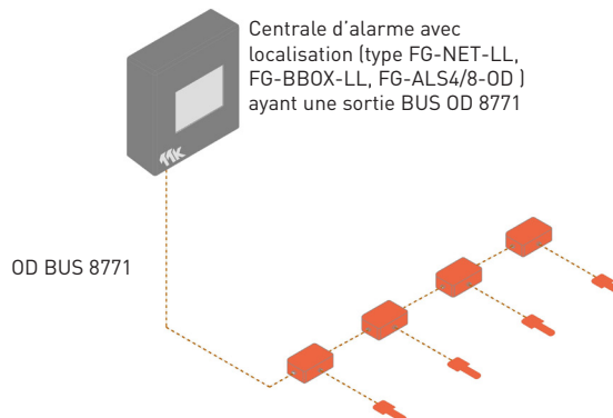
Figure 1.4.6.1 : Installation du capteur ponctuel FG-ODP sur 1 circuit d'une centrale avec localisation utilisant boîtier FG-DOP
