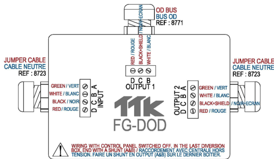
Figure 1.4.5: Schéma de câblage du boîtier d'interface FG-DOD
