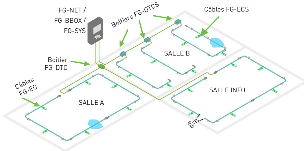
Figure 1.4.3 : Installation avec les boîtiers FG-DTC et FG-DTCS
