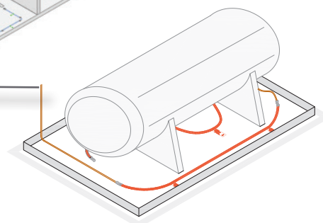
Application générateur diesel
