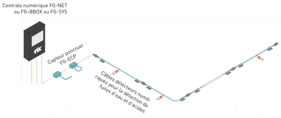
Figure 1.3.1.2: Schéma de connexion mixte des capteurs ponctuels FG-ECP et des câbles détecteurs numériques FG-EC sur un circuit de la centrale numérique FG-NET
