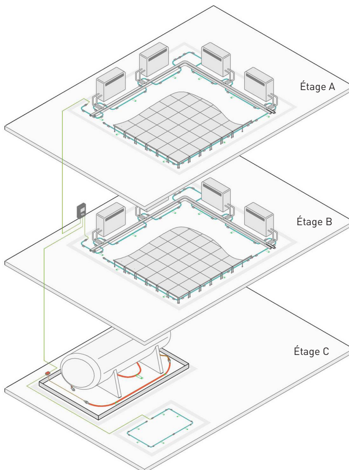
Figure 1.6 Installation « verticale »
