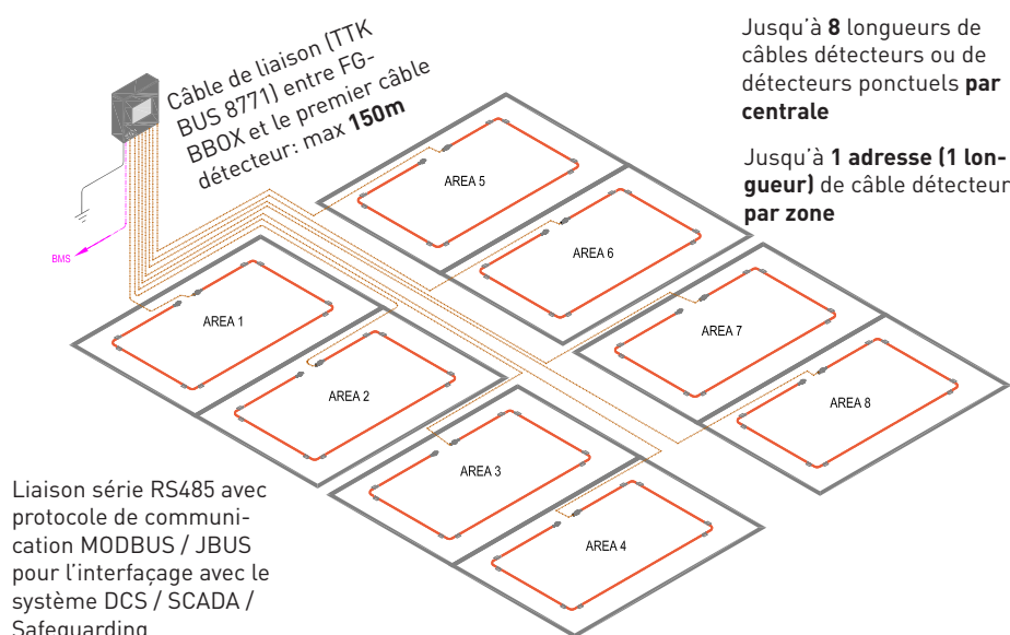
Figure 1.2.5 : Installation de FG-ALS8-OD avec 8 zones
