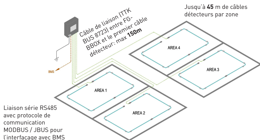
Figure 1.2.6 : Installation de FG-ALS4 avec 4 zones
