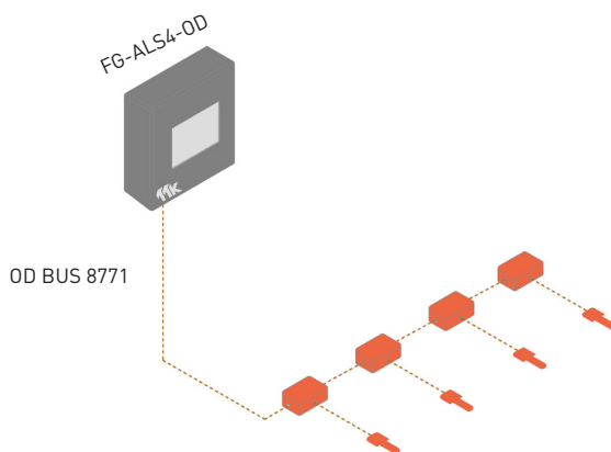
Figure 1.3.2.2: Installation du capteur ponctuel FG-ODP sur 1 circuit de la centrale FG-ALS4-OD utilisant boîtier FG-DOP
