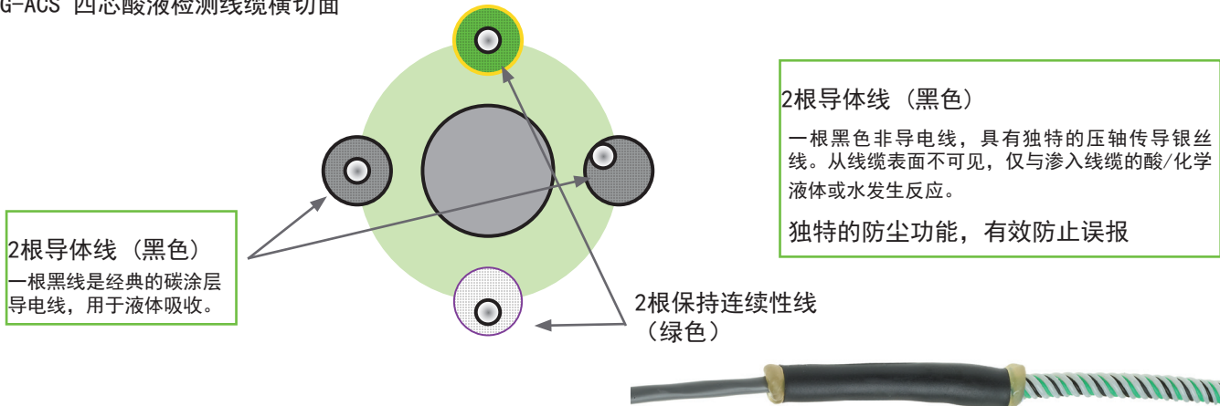
FG-ACS 四芯酸液检测线缆横切面
