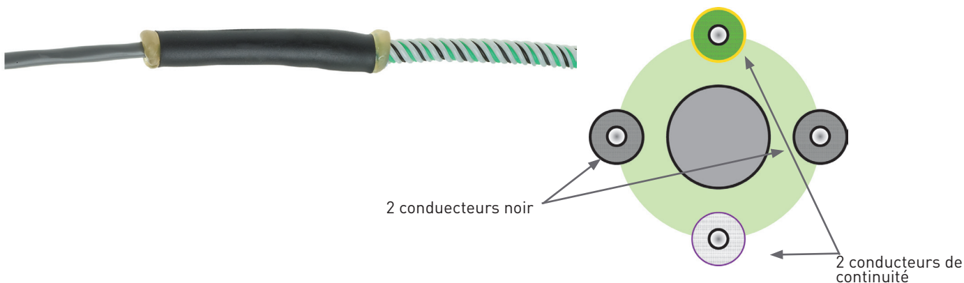
Câble détecteur FG-ACS en coupe avec ses quatre conducteurs
