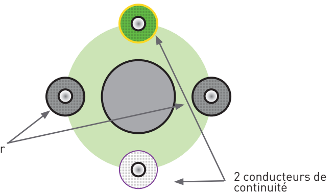
Câble détecteur FG-ACX en coupe avec ses quatre conducteurs
