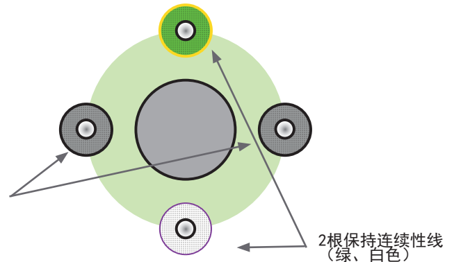
FG-ACX 4芯酸液检测线缆横切面
