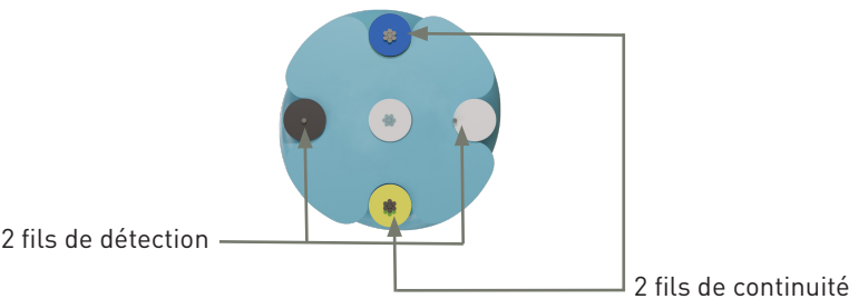
Vue en coupe du câble détecteur FG-ECX
